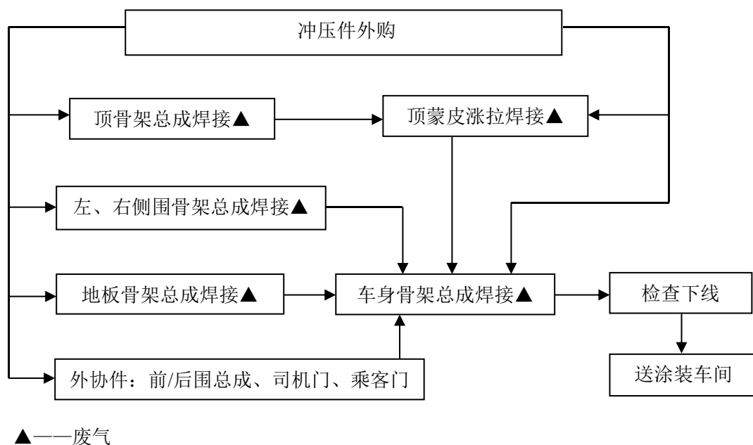
图 3.1-2 车身车间焊接工艺流程图
