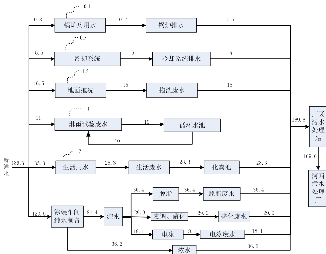
图 3.1-8 现有工程水平衡图 单位：m³/d
