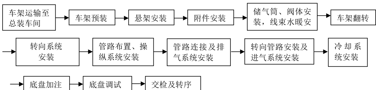
图 3.1-5 底盘装配工艺流程图
