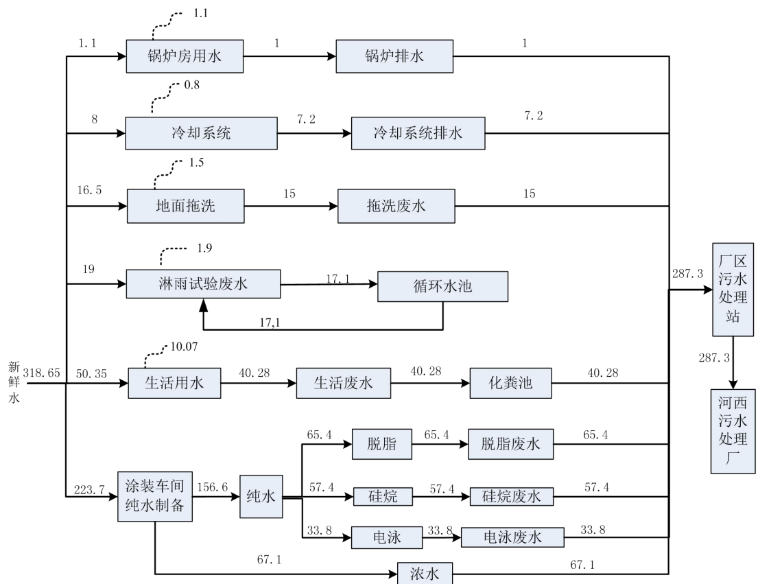
图 3.3-13 项目水平衡图 单位：m³/d
