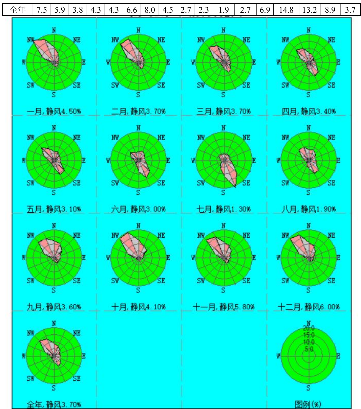
图 5.2-2 株洲市近 20 年相应风向频率玫瑰图
