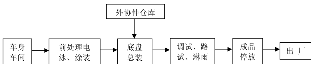
图 3.1-1 现有工程生产工艺流程图
