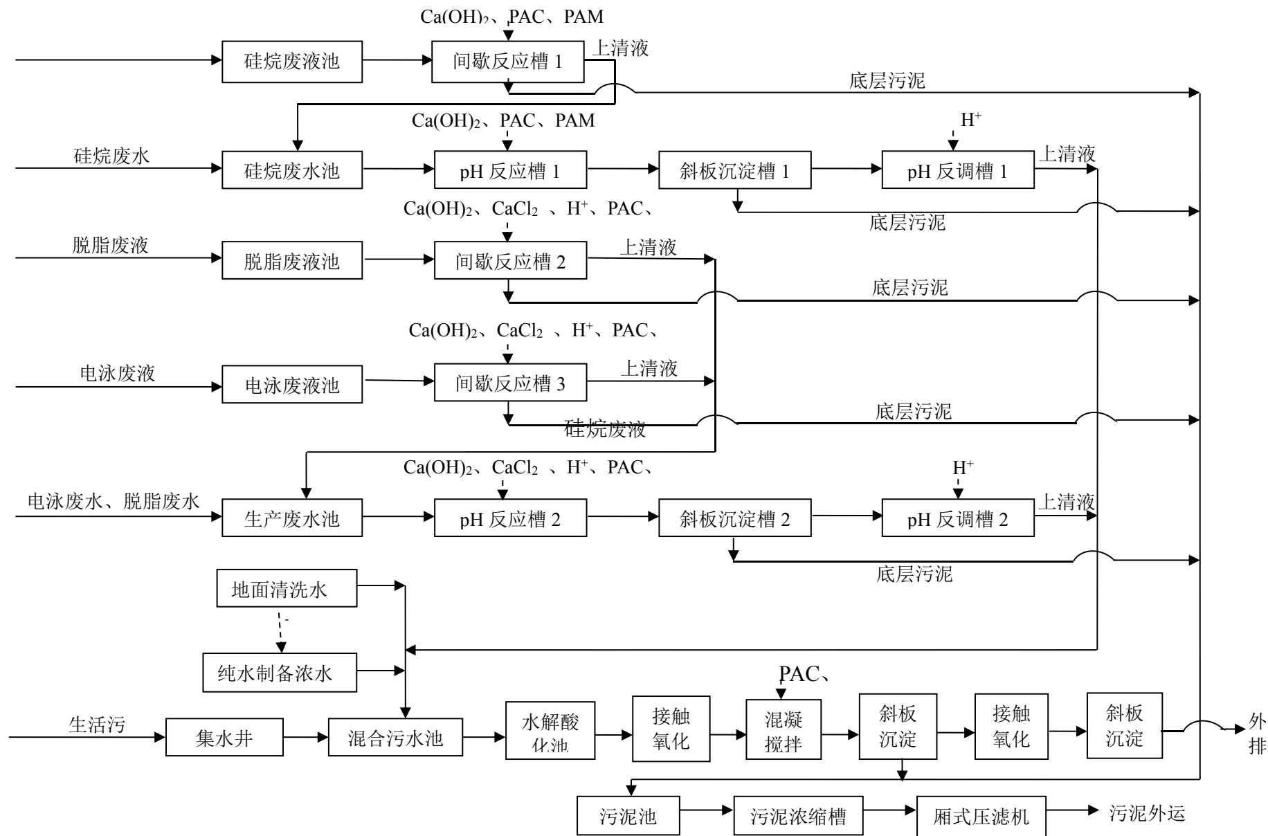
图 7.2-1 污水处理站处理工艺流程图
